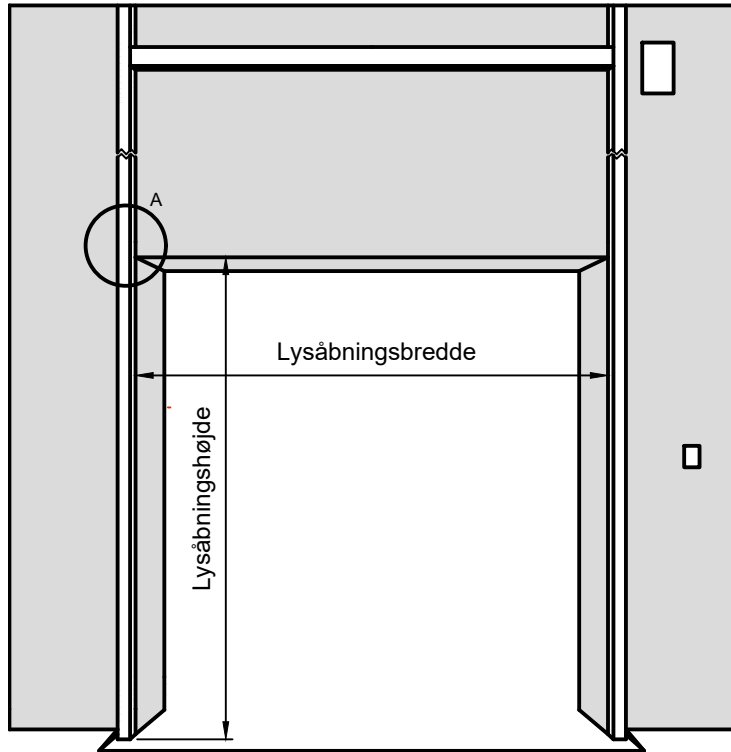
Karmløsning med 40 mm dybe lodrette karmprofiler
