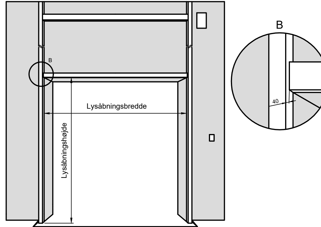
Alternativ karmløsning med 40 mm lodret/vandret karmdifference
